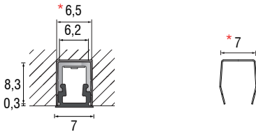
6010001 Clip di fissaggio (incluso) Fixing clip (included) Befestigungsclip (inbegriffen)
